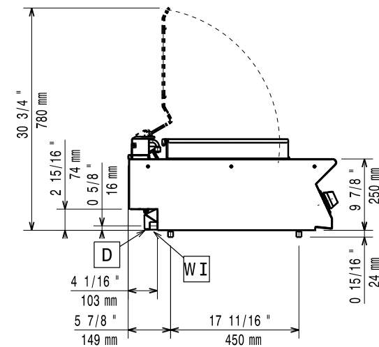
Zij aanzicht
